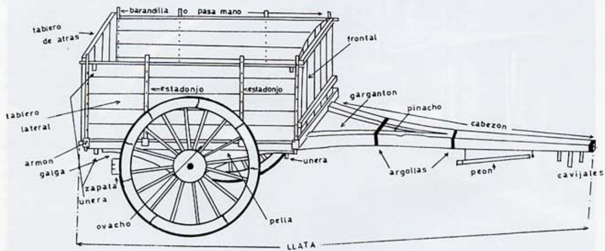
Esquema del carro.
